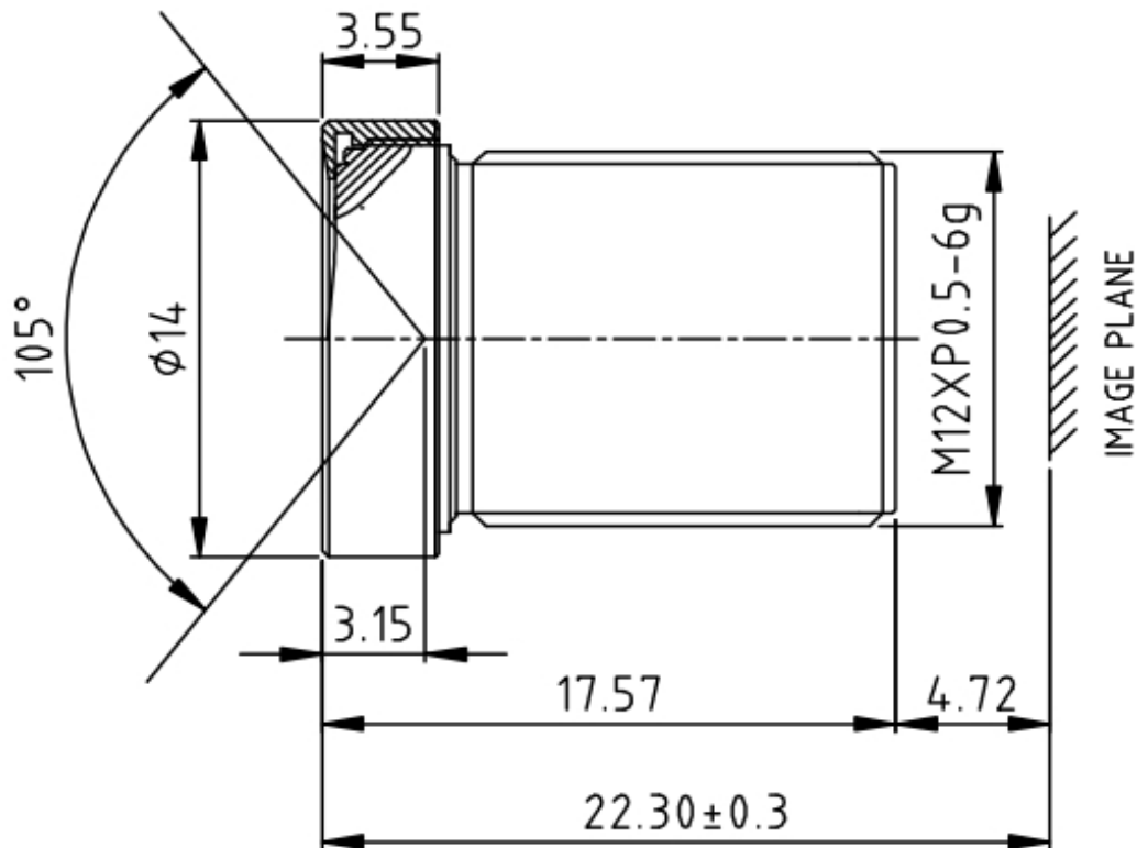
寸法図
